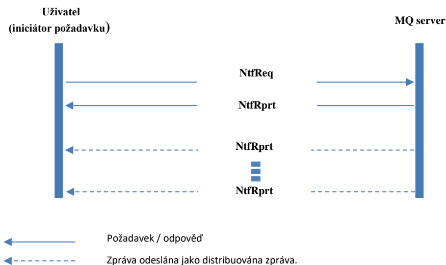
Obrázek 122 – Sekvenční schéma provedení dotazu na notifikační zprávy
