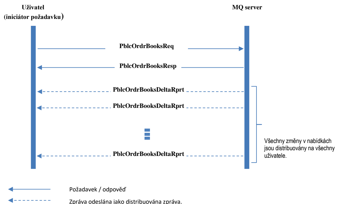
Obrázek 7 – Sekvenční schéma provedení dotazu na nabídky
