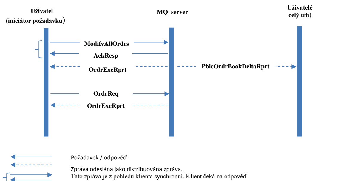
Obrázek 6 – Sekvenční schéma hromadné modifikace nabídek (deaktivace) a následný dotaz na nabídky
