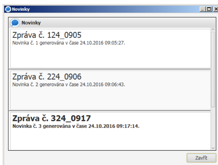
Obrázek 3 – Novinky
