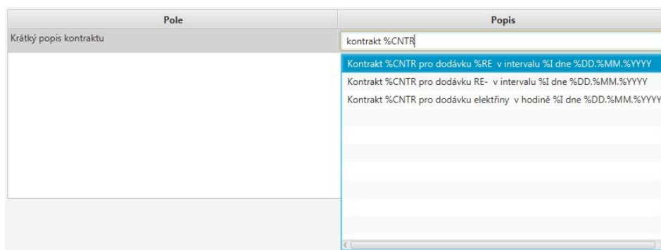
Obrázek 9 – Autocomplete box
