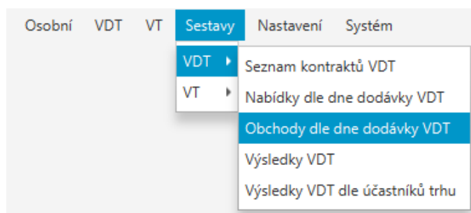
Obrázek 5 – Plovoucí menu
