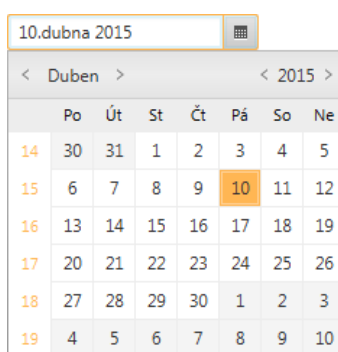
Obrázek 14 – Objekt Kalendář
