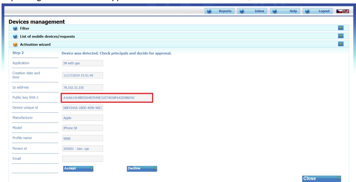
Fig. 1 –Web portal
